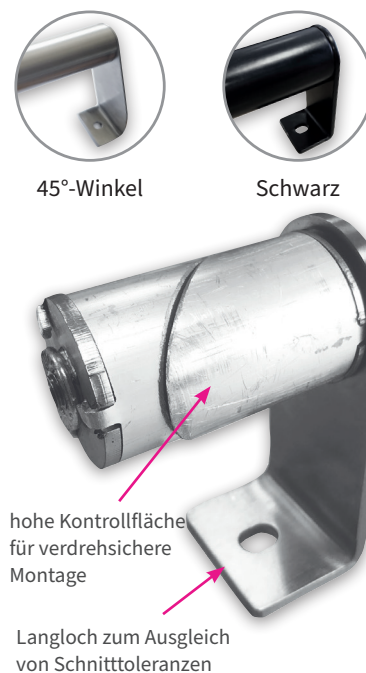
Winkelkonsole „hfb“ für Holz-Griffstange
